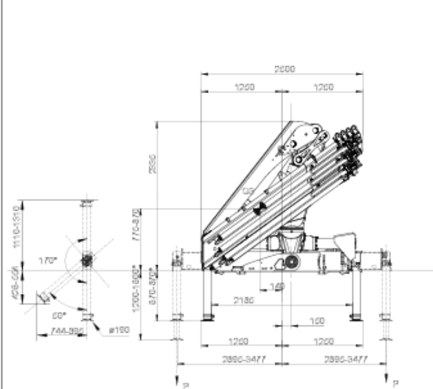
Vista frontal con el brazo retraído
