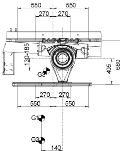
Instalación del chasis
